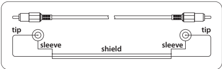
Fig. 4.5: RCA cable
